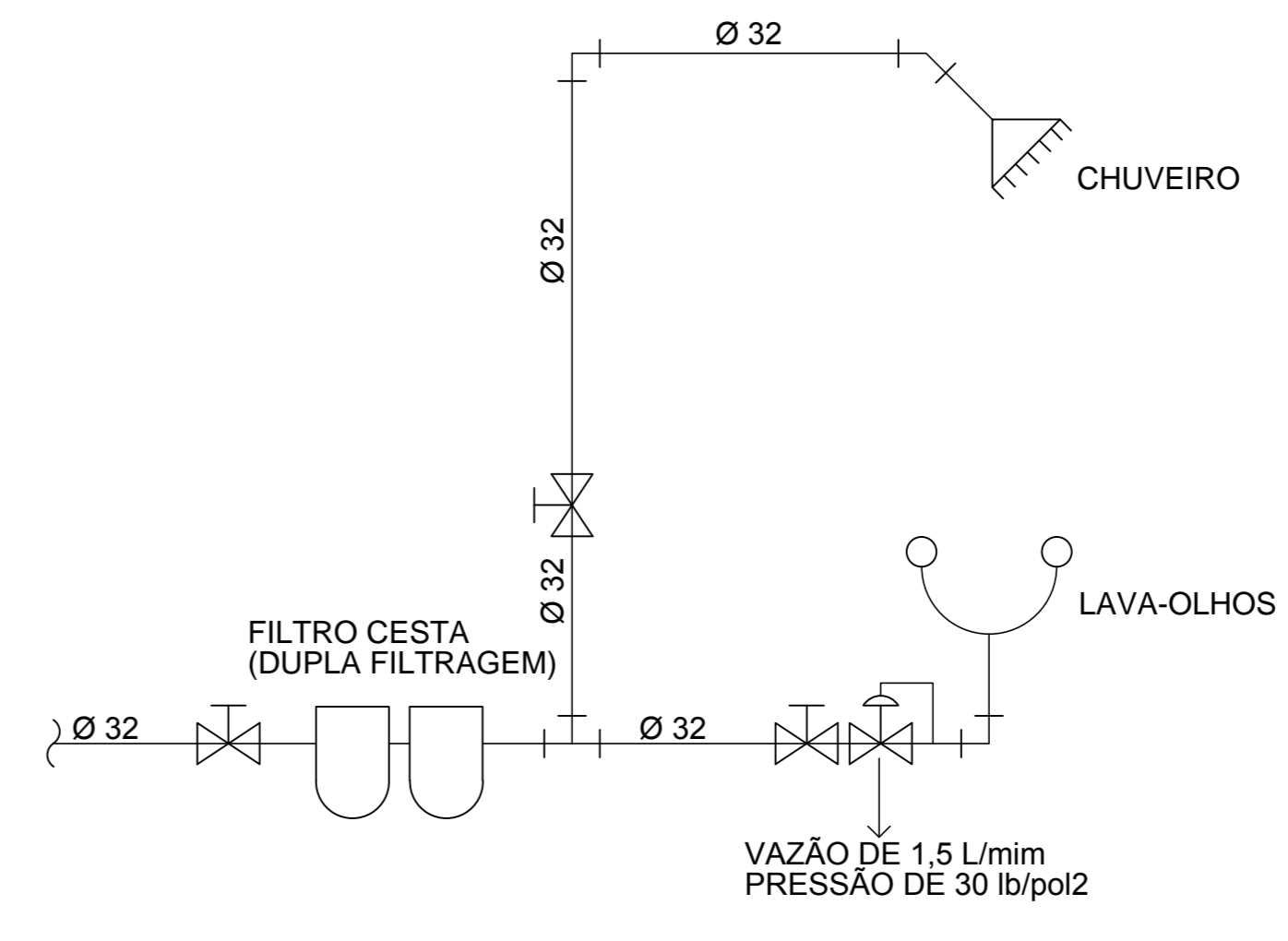
08 DETALHE LAVA-OLHOS SEM ESCALA
