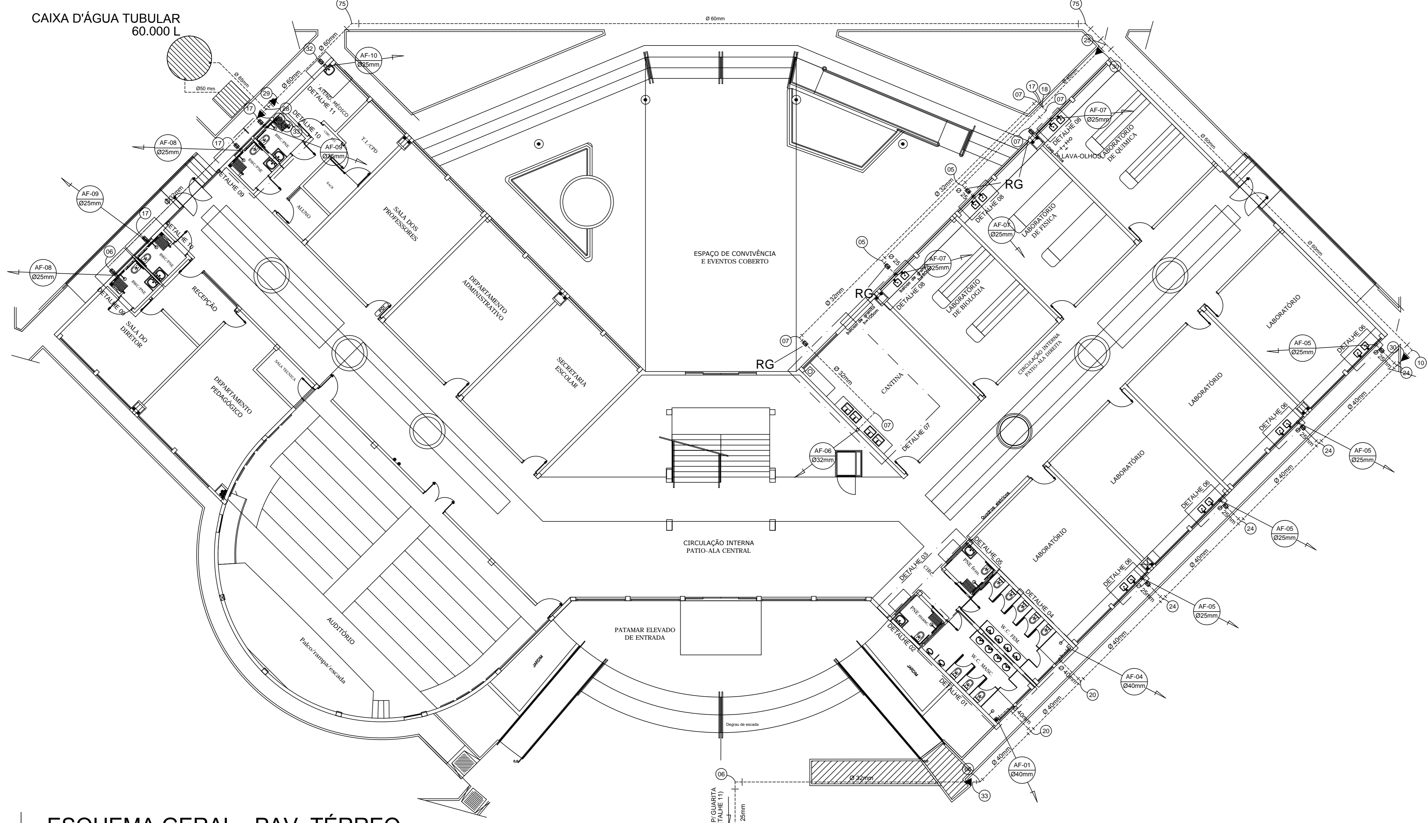
04 ESQUEMA GERAL - PAV. TÉRREO ESCALA 1 : 125
