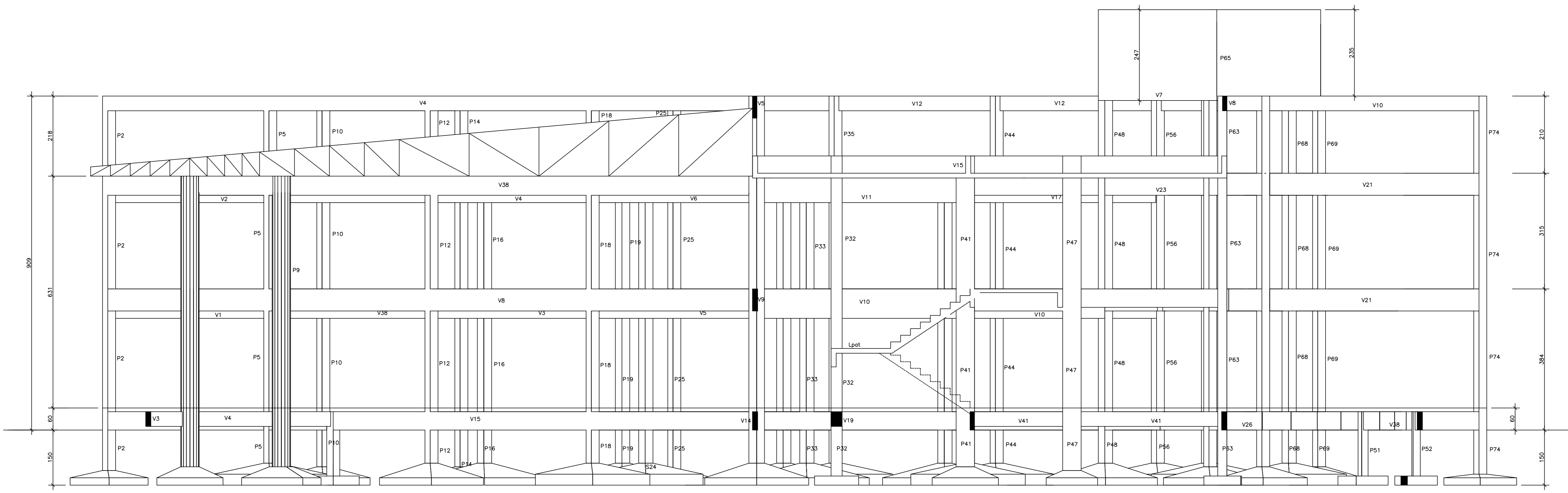
Corte B-B Escr: 1/50
