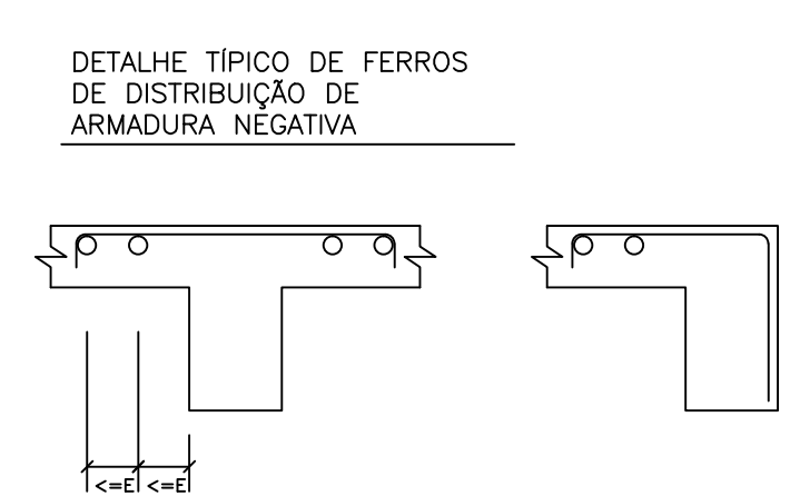
Piso - Armadura negativa vertical Esc: 1/25
