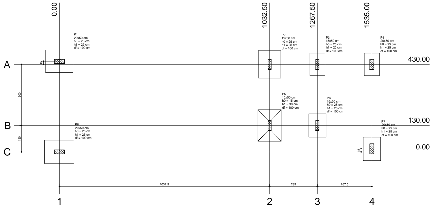
Planta de locação escala 1:50
