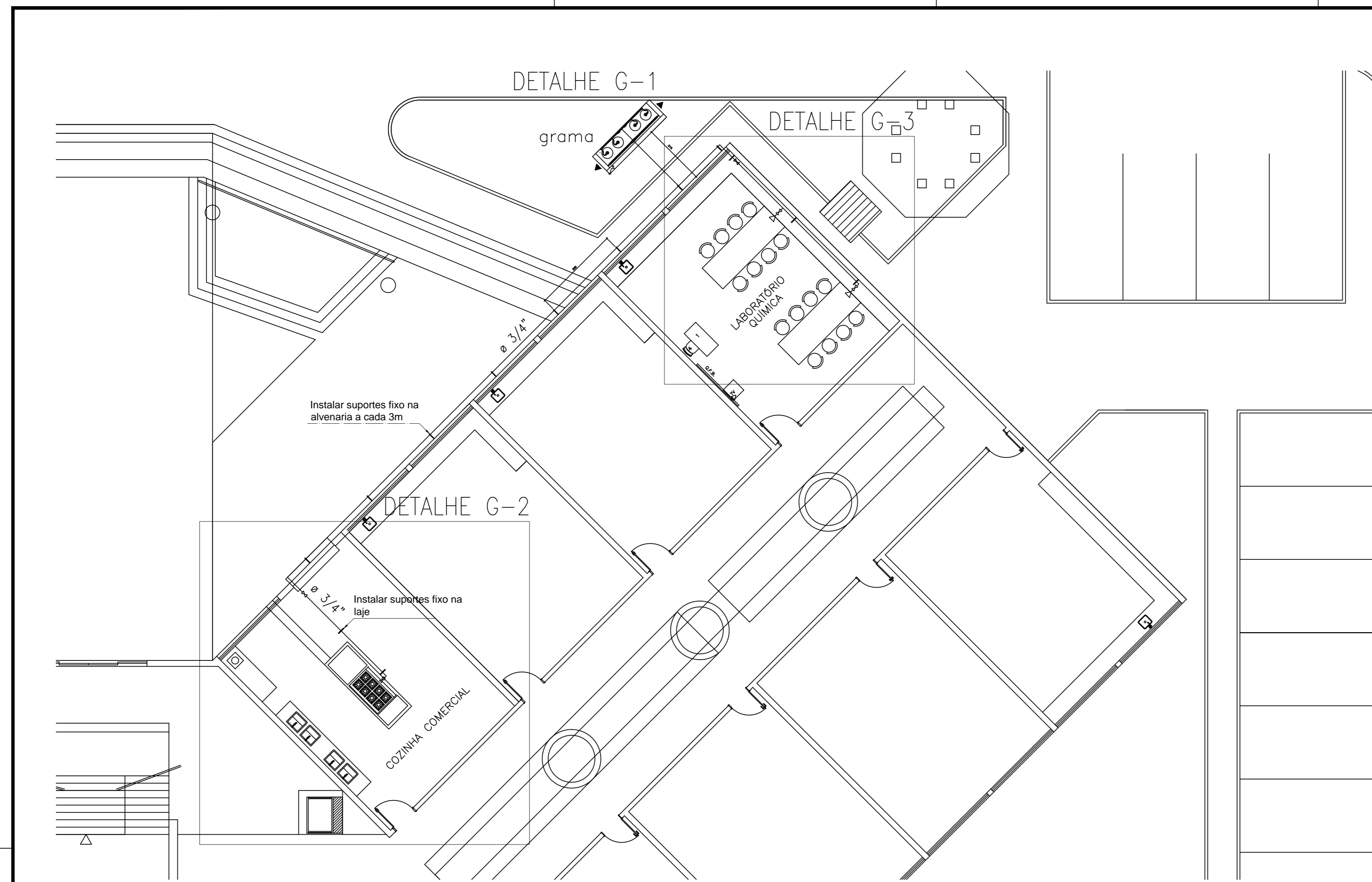
01 PLANTA BAIXA ESCALA: 1:100
